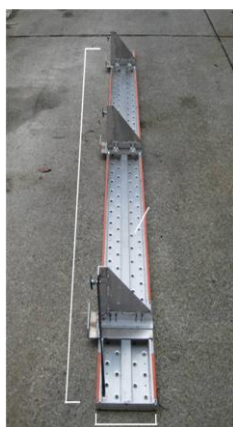
<あおりに取り付ける簡易作業床の例> (荷役安全設備マニュアル (パンフレット) より)
